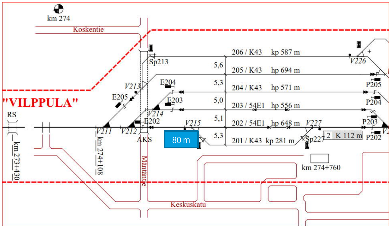
Kuva 1: Vilppulan raiteistokaavio
